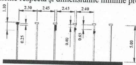
Figura 5.2 Parcarea la 90° alăturată unor elemente de construcţie poziţionate la o distanţă cuprinsă între 0 şi 1.10 m faţă de marginea căii de circulaţie
