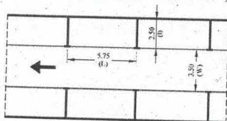
Figura 6.3 Parcarea pentru autoturisme longitudinală, la bordură, cu cale de acces cu sens unic
