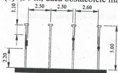
Figura 5.3 Parcarea la 90° alăturată elementelor de construcţie poziţionate la o distanţă cuprinsă între 1.10 m şi 2.80 m faţă de marginea căii de circulaţie
